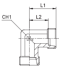
Type: 1038...1 Body
